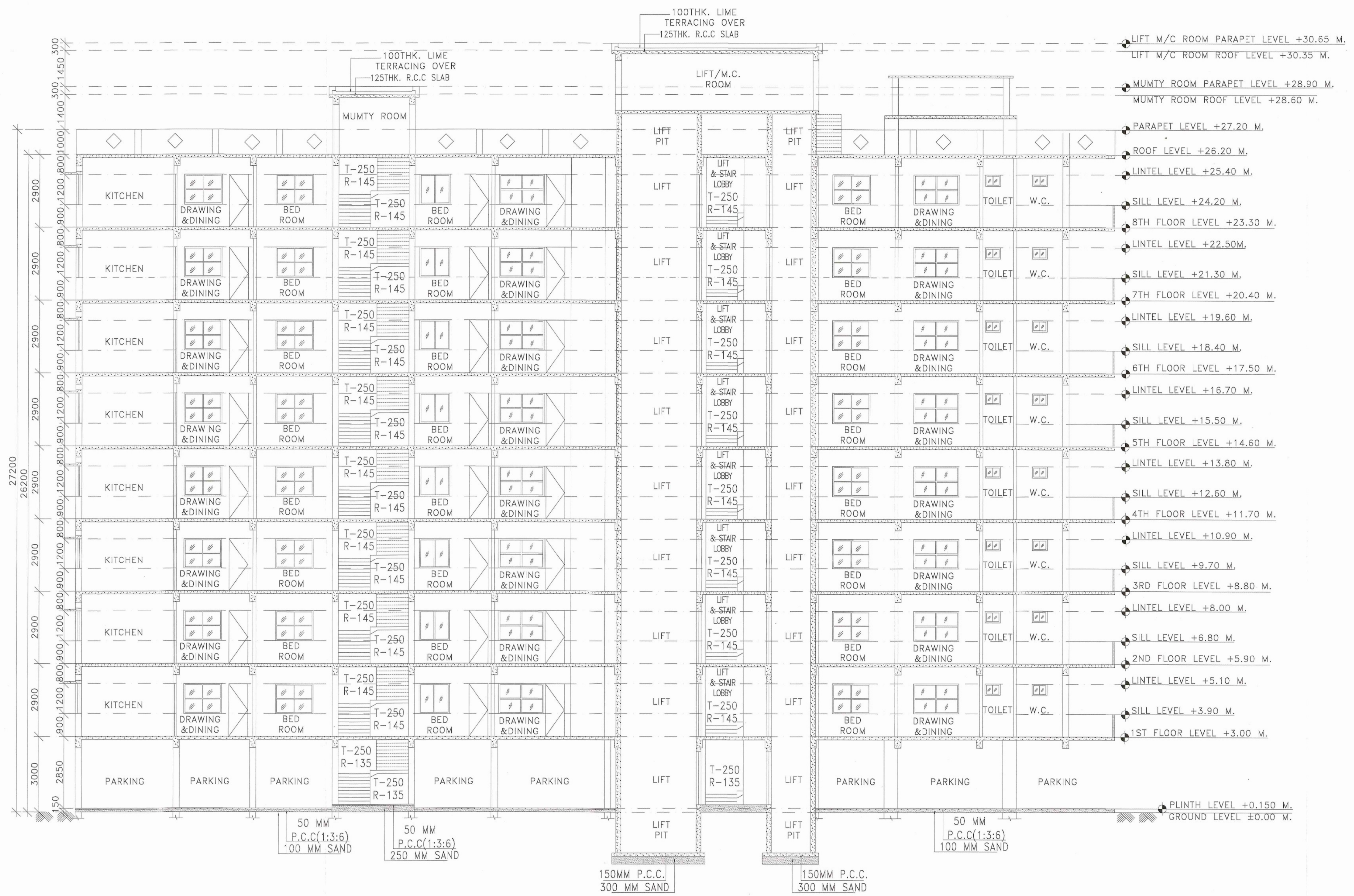
SECTION Y-Y' SCALE: 1:100
